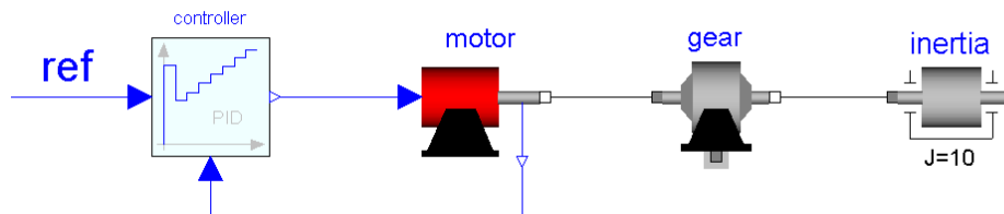
Bild 2: Objektdiagramm eines einfachen Antriebsstrangs
